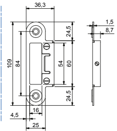
Verstelbare Loopsluitplaat Dagschoot Art. nr. 706420 (Korte Lip) (Short) Art. nr. 706430 (Lange Lip) (Long) Adjustable strike for Latchbolt Verst. Sluitpl. Automatic Dagschoot Art. nr. 706440 (Korte Lip) Adjustable Strike for Automatic Latchbolt (Short)
