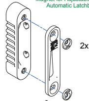
Sluitkom Dagschoot Art. nr. 707021 Casing for Adjustable Strike Latchbolt Magneet t.b.v. Automatic Dagschoot Art. nr. 200089 (6 mm) Art. nr. 200179 (10 mm) Magneet for Adjustable Strike Automatic Latchbolt
