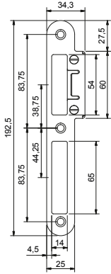
Verstelbare Sluitplaat Dag- en Nachtschoot Art. nr. 706380 (Korte Lip, Din Ls) Art. nr. 706390 (Korte Lip, Din Rs) Art. nr. 706400 (Lange Lip, Din Ls) Art. nr. 706410 (Lange Lip, Din Rs) Adjustable Strike (Short, Long) for Main Lock Case
