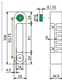
Sluitkom Dagschoot Art. nr. 707021 Casing for Adjustable Strike Latchbolt Magneet t.b.v. Automatic Dagschoot Art. nr. 200089 (6 mm) Art. nr. 200179 (10 mm) Magneet for Adjustable Strike Automatic Latchbolt
