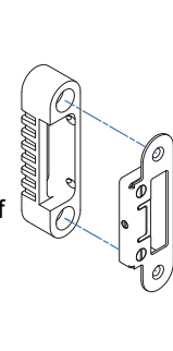
Verstelbare Loopsluitplaat Dagschoot Art. nr. 706420 (Korte Lip) (Short) Art. nr. 706430 (Lange Lip) (Long) Adjustable strike for Latchbolt Verst. Sluitpl. Automatic Dagschoot Art. nr. 706440 (Korte Lip) Adjustable Strike for Automatic Latchbolt (Short)
