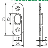
Magneet voor MPS (Auto)Motortronic Art. nr. 200076 Magneet for MPL's (Auto)Motortronic
