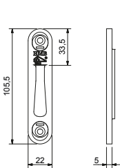
Verstelbare Sluitplaat Haakschoot Art. nr. 600357 Adjustable Strike for Hookbolt
