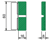
Verlengblokje voor Verst. Sluitpl. Art. nr. 600599 (16 mm) Art. nr. 600598 (12 mm) Art. nr. 600597 (8 mm) Art. nr. 600596 (4 mm) Strike Extenders (size)
