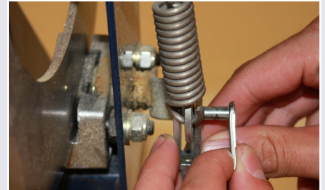
Afb. 12 Verbinden remschaar
