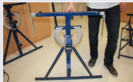
Afb. 3 Zijkant
