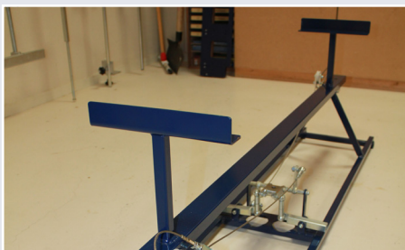
Afb. 1 Basisframe
