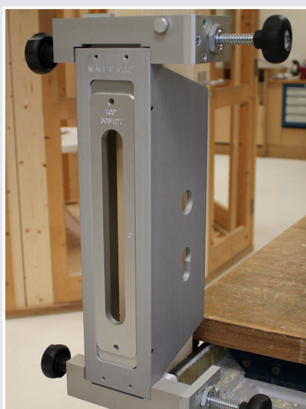
Afb. 13 Moedermal incl. U-cassette en
