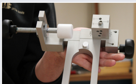
Afb. 4 Moedermal met 5 mm vulpropje (DM 55)
