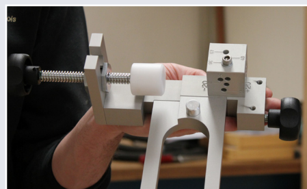
Afb. 5 Moedermal met 10 mm vulpropje (DM 50)
