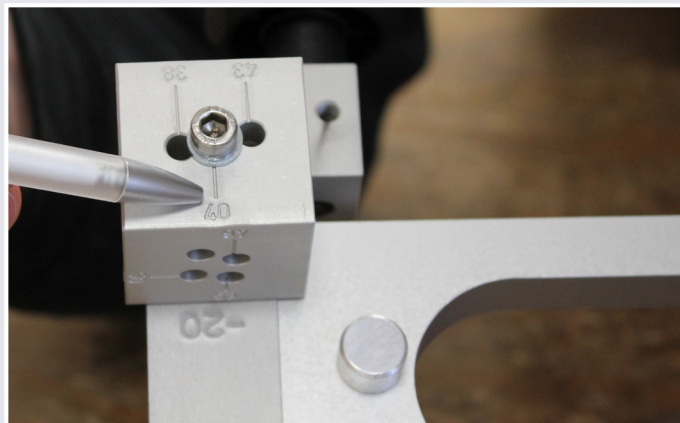
Afb. 9 Positie Maatkubus op Moedermal
