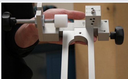
Afb. 3 Moedermal zonder vulpropje (DM 60)
