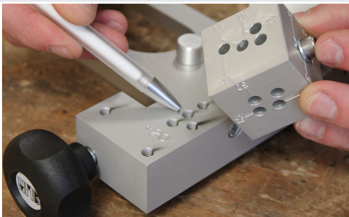
Afb. 8 Maatkubus plaatsen op Moedermal
